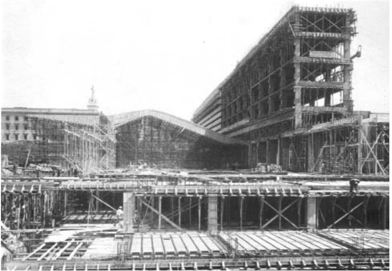
Costruzione dell'edificio di testa e dell'atrio biglietteria (il "Dinosauro"), 1949
