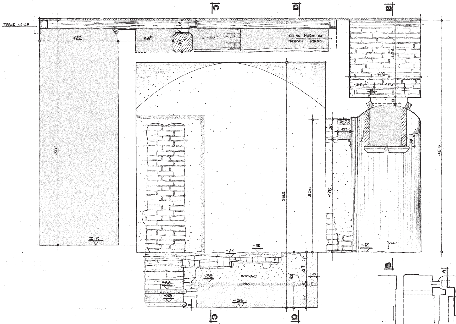
SEZIONE A-A VEDERE ANCHE LE SEZIONI BB, CC, DD
