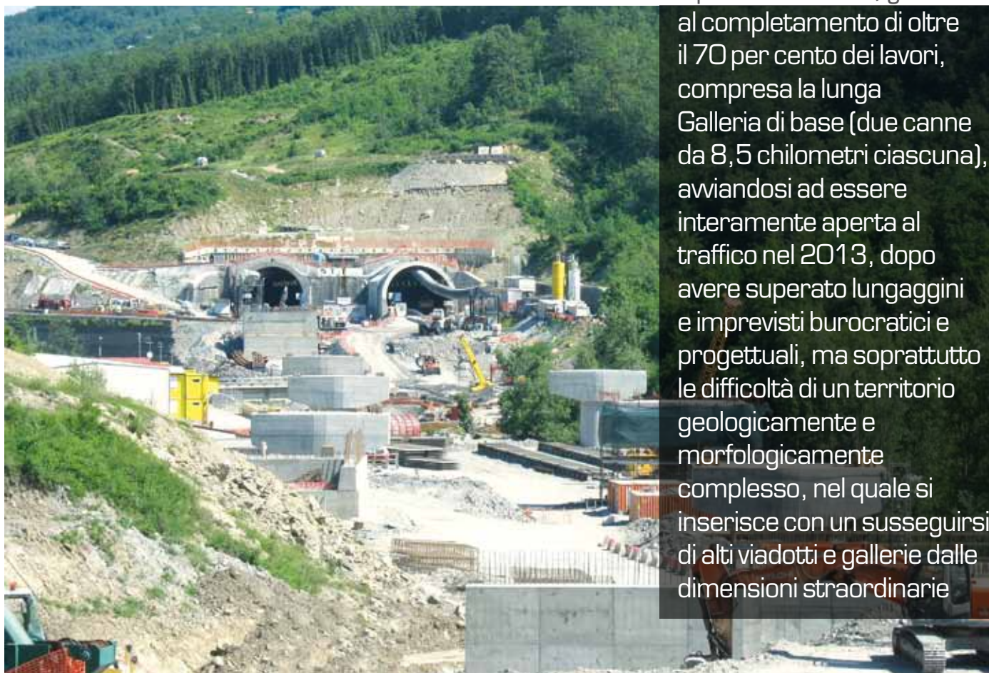
Veduta del viadotto Sparvo e dell'imbocco lato Firenze della galleria Val di Sambro, una delle più complesse del lotto 6-7 della Variante di Valico, fra le ultime ad essere completata
